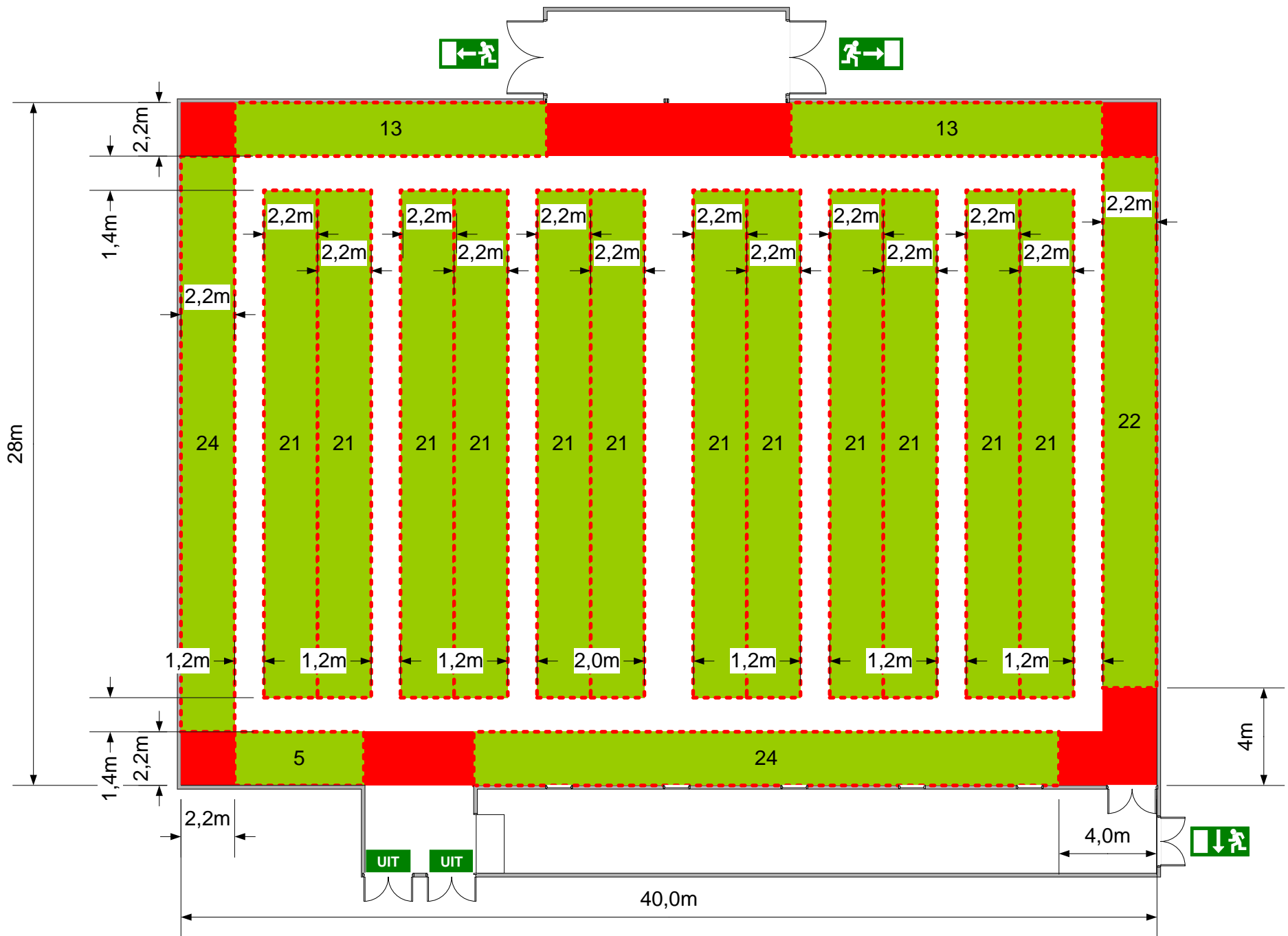
Sporthal 1 – Schaal 1:200 – Maximaal 353 personen
