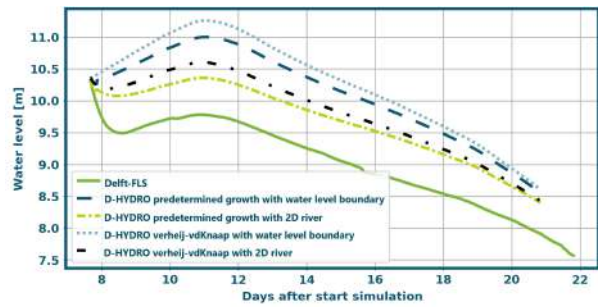
(D) Upstream water level at Tiel
