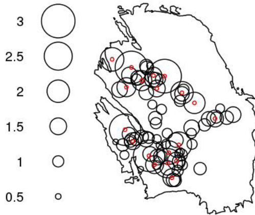
LEGENDA: Cirkels rond epicentra van aardbevingen in het Groninger veld gedurende 2014 en met straal recht evenredig aan de magnitude. Bevingen met magnitude 1,5 of zwaarder zijn in het rood weergegeven. Deze gegevens worden bijgehouden op het portaal [18].
