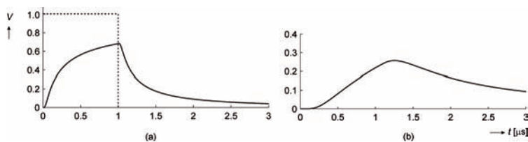
Figuur 2: Respons van een telefoonlijn op een data-sigitaal; lengte 1 \text{ km} (a) en lengte 3 \text{ km} (b)
