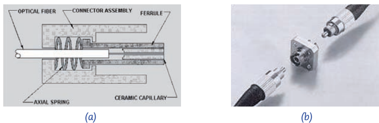
Figuur 7: Doorsnede van een optische connector (a); connectoren met koppelstukje (b)
