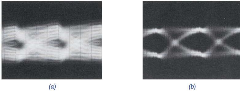
Figuur 5: Data-sigitaal zoals dat getransporteerd is over 1 km kabel (a); na correctie van de storingen (b)
